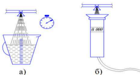
Сурет 2. Бүріккіштердің шығыс сипаттамаларын анықтау а) өлшеуіш цилиндр және секундомер көмегімен; б) экспресс-тестердің көмегімен;
