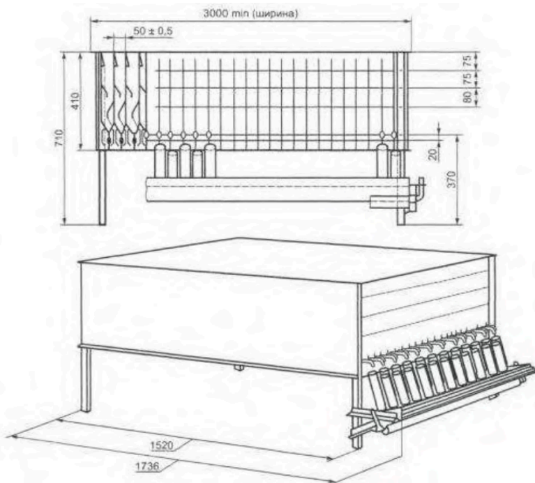
Сурет 6. Тозаңдату жабдығын сынау кезінде сынау стендінің үлгі түрі (MEMCT ISO 5682-1-2004 алынды)
