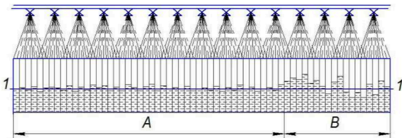
Сурет 4. Бүріккіштің басып алу ені бойынша жұмыс сұйықтығының біркелкі бөлінбеуін анықтау
