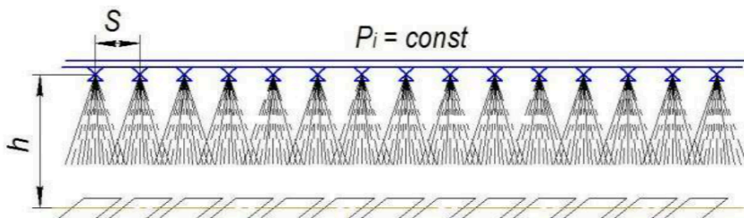
Сурет 5. Бүріккіштің тарату жүйесіне далалық сынақтар жүргізу кезінде ұстап қалатын беттерді орналастыру
