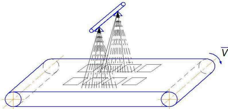
Сурет 7. Бүріккіш штангасының ленталы транспортердің көмегімен өңделетін беттің үстінен қозғалуын имитациялау
