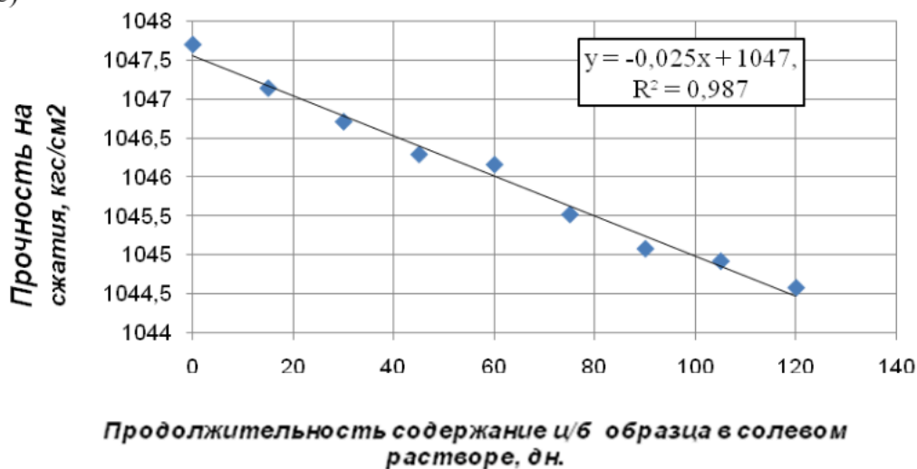
Рис. 2. Потеря прочности цементобетонных образцов в соевых растворах:
