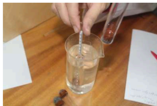
Рисунок 1 – Определение концентрации растворов противогололедных реагентов:
